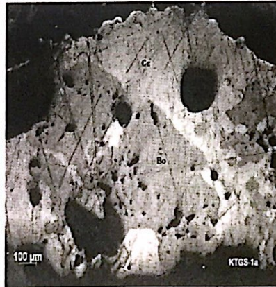
Ảnh 5. Chalcocin (Cc) và bornit (Bo) tạo đám ổ xâm tán trên nền phi quặng
