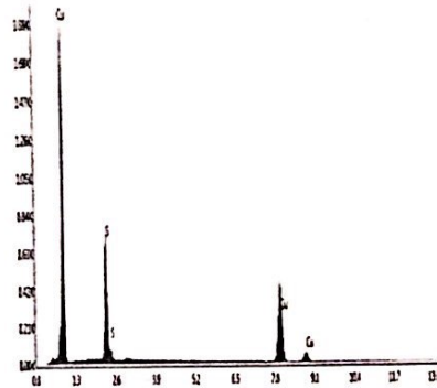
H.3. Kết quả phân tích SEM tại EDS spot 2-Khoáng vật chalcocin
