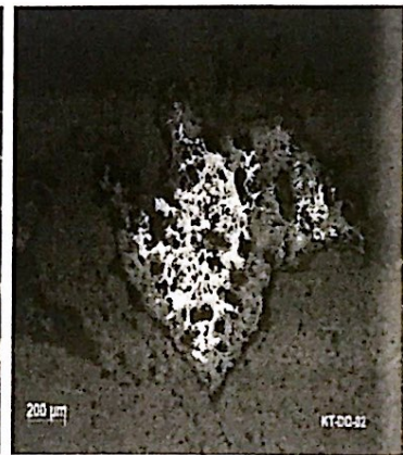
Ảnh 6. Covenlin (Cv) tạo vành riềm bao quanh tennantit (Te)
