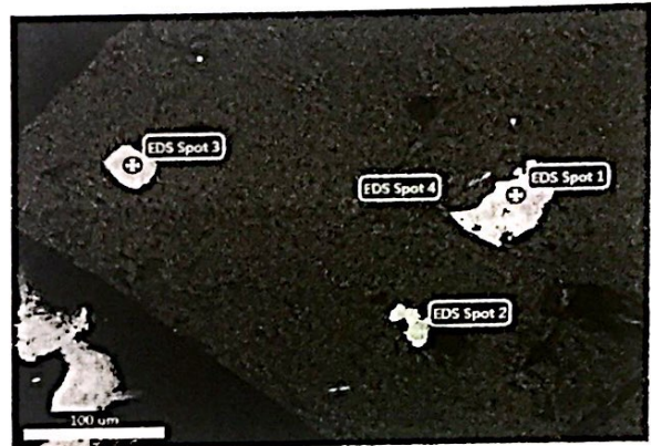
Ảnh 14. Các khoáng vật mẫu KTGS 23/2 chụp dưới kính hiển vi điện tử quét SEM và các điểm xác định thành phần các nguyên tố khoáng vật
