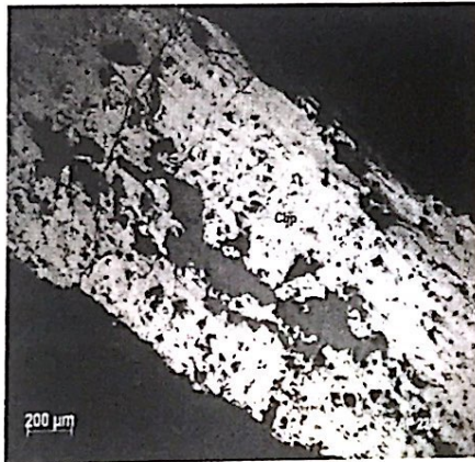
Ảnh 4. Chalcopyrit (Chp) và tennantit (Te) tạo mạch lấp đầy trong các vi khe nứt
