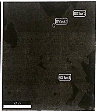
Ảnh 12. Điểm bắn các khoáng vật mẫu KT-17 chụp dưới kính hiển vi diện tử quét SEM
