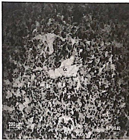
Ảnh 8. Bornit (Bo) và chalcocin (Cc) xâm tán dày trên nền phi quặng
