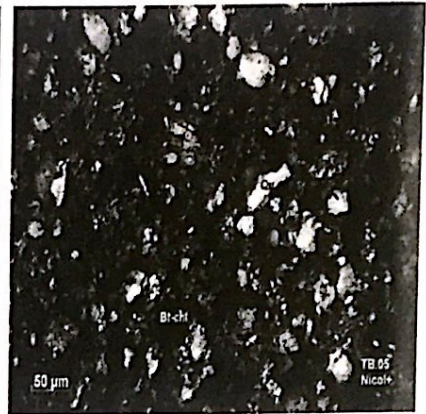
Ảnh 3. Các tấm vẩy biotit trong bột kết đa khoáng bị chlorit hóa mỏ Trại Bấu. cl-clorit; Qu (quặng); Pl - plagioclaz
