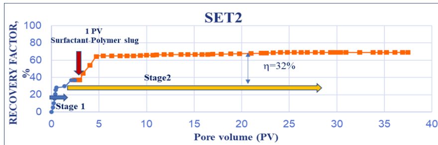
Fig. 4. Core flooding results of the second core plug set Rys. 4. Wyniki drugiego zalania rdzenia
