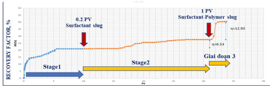
Fig. 3. Core flooding results of the first set core plug Rys. 3. Wyniki pierwszego zalania rdzenia
