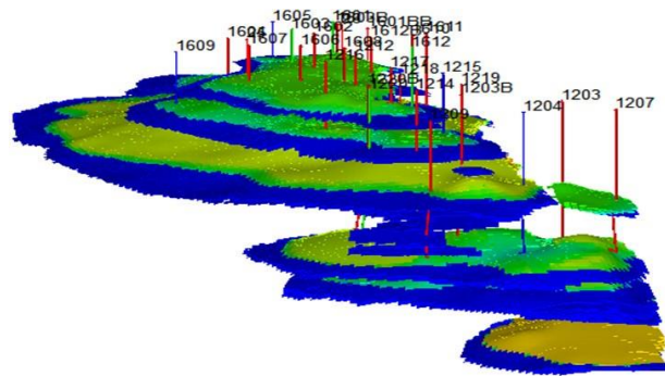
Fig. 5. Simulation model of Lower Miocene, Southern dome, field Bach Ho Rys. 5. Model symulacyjny Dolny Miocen, kopuła południowa, pole Bach Ho
