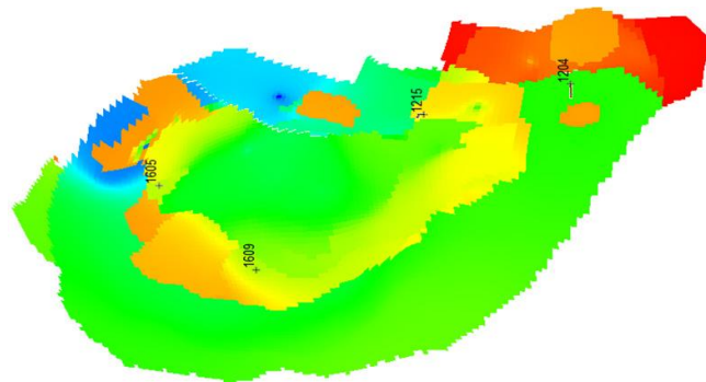
Fig. 6. Location of injection wells on the simulation model of Lower Miocene, Southern dome, Bach Ho field Rys. 6. Lokalizacja odwiertów zatłaczających na modelu symulacyjnym złoża Dolny Miocen, kopuła południowa w polu Bacha Ho
