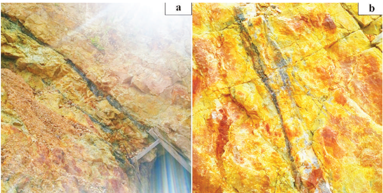
H.6. Một số hình ảnh thể hiện các mạch quặng và đới biến đổi đi kèm tại mong khai thác và lỗ khoan (PDD-19) khu vực Phu Dao, mỏ vàng Sakai. a,b- Các thân quặng vàng dạng mạch, mạng mạch trong đá tuf ryolit
