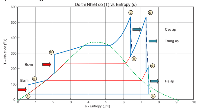
Hình 3. Chu trình Clausinus-Rankine Nhà máy nhiệt điện Đồng Triều.
