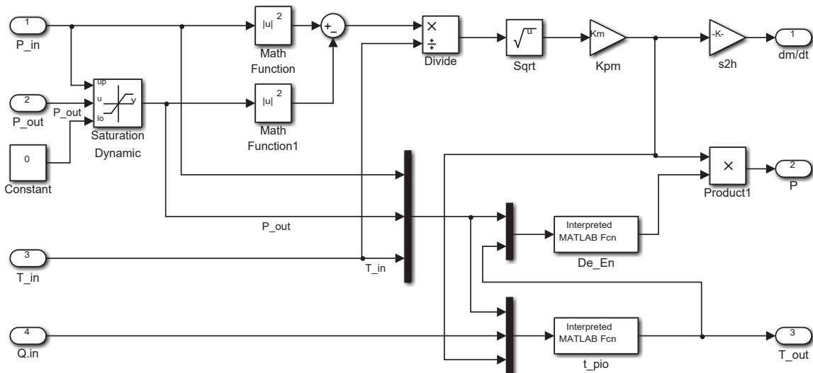
H.4. Cấu trúc mô phỏng lưu lượng khối – áp suất
