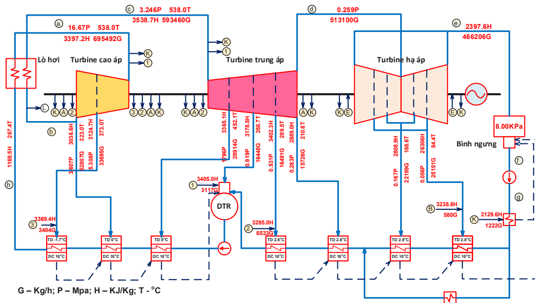
Hình 1. Sơ đồ nhiệt nguyên lý của nhà máy nhiệt điện Đông Triều.
