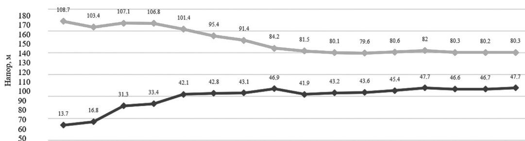
Рис. 6. Пьезометрический график от теплового источника до распределительной тепловой камеры после устройства новой ПНС
