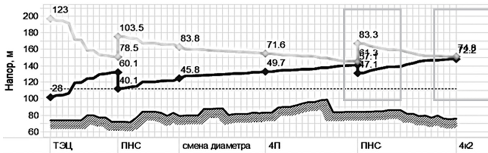
Рис. 3. Пьезометрический график от теплового источника до распределительной тепловой камеры до реконструкции существующей ПНС Fig. 3. Piezometric diagram from the heat source to the heat distribution chamber before the reconstruction of the existing booster pumping station
