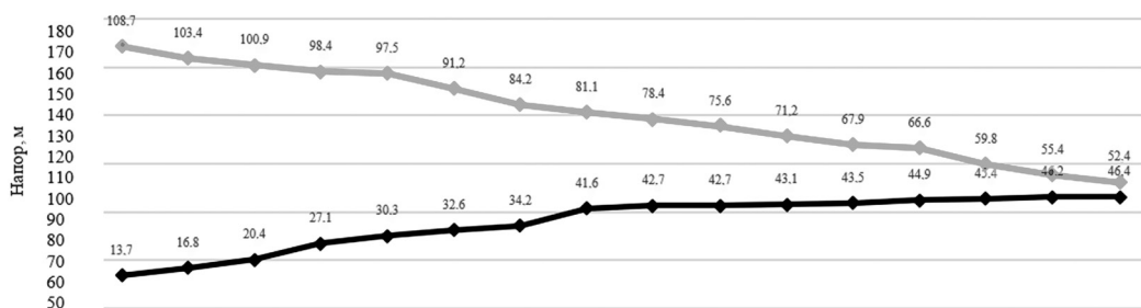
Рис. 5. Пьезометрический график от теплового источника до распределительной тепловой камеры до устройства новой ПНС
