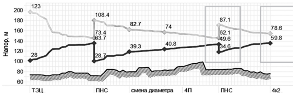
Рис. 4. Пьезометрический график от теплового источника до распределительной тепловой камеры после реконструкции существующей ПНС Fig. 4. Piezometric diagram from the heat source to the heat distribution chamber after the reconstruction of the existing booster pumping station
