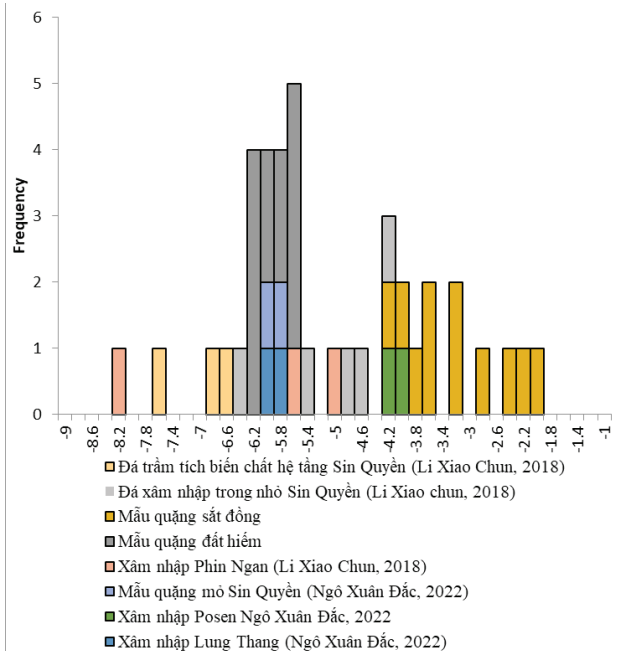
H.9. Biểu đồ giá trị \epsilon_{\text{Nd}}(t) hai loại titanite và các thể xâm nhập felsic, đá trầm tích biến chất trong khu vực và mỏ Sin Quyên
