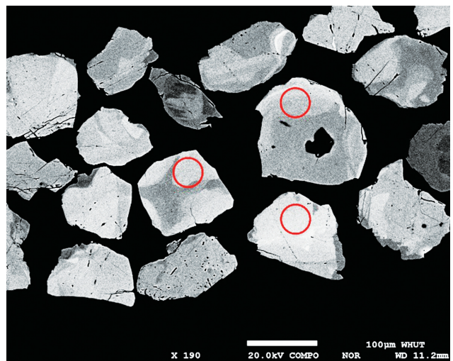
H.8. Phân tích SEM xác định điểm bản đồng vị Nd đối với titanit thành tạo giai đoạn hai.
