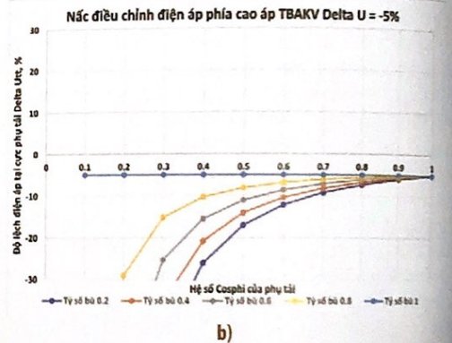
H.1. Quan hệ phụ thuộc giữa \Delta U_{tt} với hệ số công suất \cos\varphi của phụ tải và tỷ số bù K , theo các cấp điều chỉnh điện áp phía cao áp TBAKV
