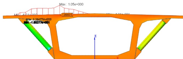
(a) Mặt bằng ứng suất trong trường hợp có thanh chống a = 3\text{m} .
