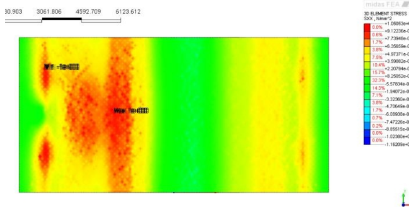
(a) Mặt bằng ứng suất trong trường hợp có thanh chống a = 3\text{m} .
