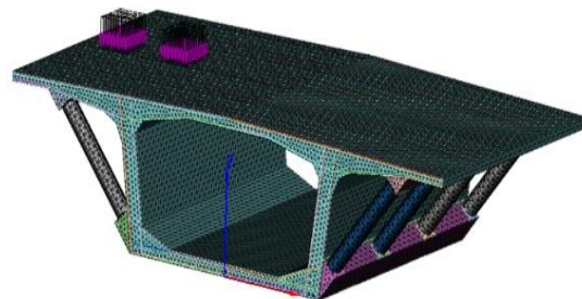
(b) Thanh chống với a = 2 \text{ m} .
