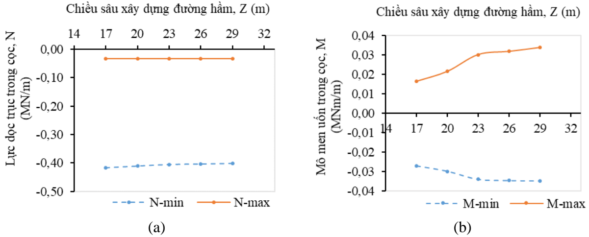
Hình 13: Mối tương quan giữa lực dọc trục trong cọc (a), mô men uốn trong cọc (b) với chiều sâu xây dựng đường hầm: Z=17m; Z=20m; Z=23m; Z=26m; Z=29m
