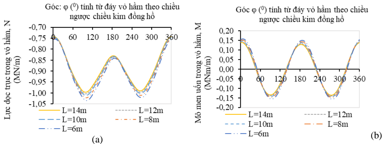
Hình 9: Lực dọc trục trong vỏ hầm (a), mô men uốn trong vỏ hầm (b) đối với khoảng cách từ trục đường hầm đến cọc: L=14\text{m} ; L=12\text{m} ; L=10\text{m} ; L=8\text{m} ; L=6\text{m}
