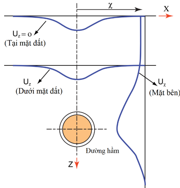
Hình 3: Đường cong dịch chuyển lớp đất xung quanh đường hầm, Simpson et al. (1996) [12]
