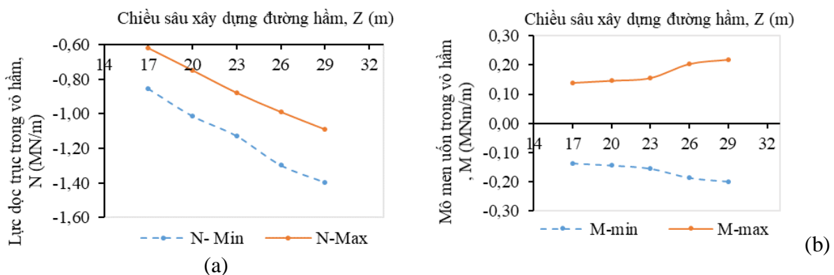
Hình 12: Mối tương quan giữa lực dọc trục trong vỏ hầm (a), mô men uốn trong vỏ hầm (b) với chiều sâu xây dựng đường hầm: Z=17m ; Z=20m ; Z=23m ; Z=26m ; Z=29m
