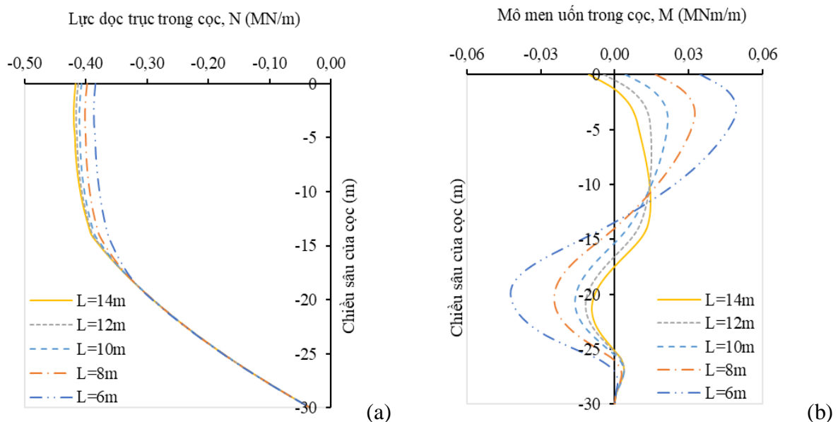
Hình 10: Lực dọc trục trong cọc (a), mô men uốn trong cọc (b) đối với khoảng cách từ trục đường hầm đến cọc: L=14\text{m} ; L=12\text{m} ; L=10\text{m} ; L=8\text{m} ; L=6\text{m}
