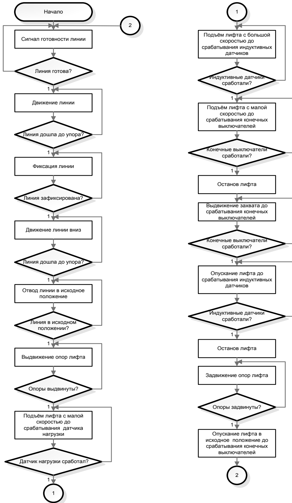
Рисунок 1 – Алгоритм работы комплекса лифтовой транспортировки кузова автомобиля
