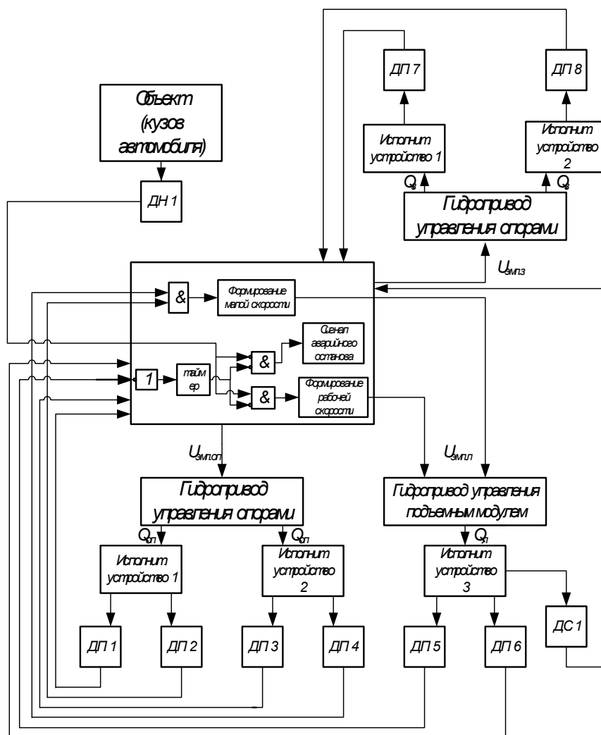
Рисунок 2 – Функциональная схема электрогидравлической системы управления
