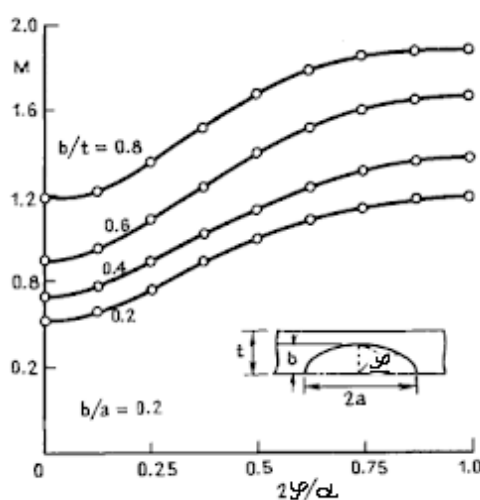
Рисунок 1 – Зависимость КИН от глубины и ширины повреждения.
