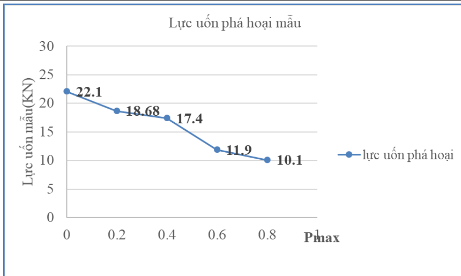
Hình 11. Biểu đồ quan hệ ứng suất và lực phá hoại mẫu
