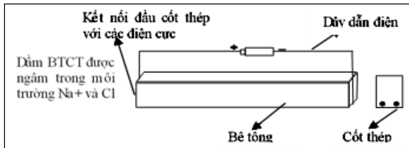
Hình 3. Mô tả thiết bị gông mẫu dầm thực nghiệm
