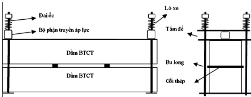
Hình 3. Mô tả thiết bị gông mẫu dầm thực nghiệm
