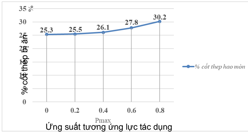
Hình 9. Biểu đồ quan hệ lực tác dụng và tốc độ ăn mòn
