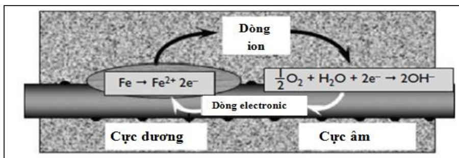
Hình 4. Mô hình diễn tiến nhanh ăn mòn điện cực mẫu dầm thực nghiệm
