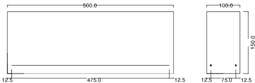
Hình 1. Hình dạng và cấu tạo dầm thí nghiệm
