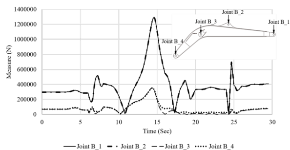
Fig. 8. Joint reaction forces of boom Rys. 8. Siły reakcji bomu na przegub
