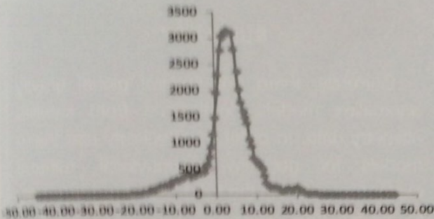
H.2. Biểu đồ tần suất xuất hiện của độ lệch giữa DTU10GRAV so với số liệu đo trực tiếp bằng tàu
