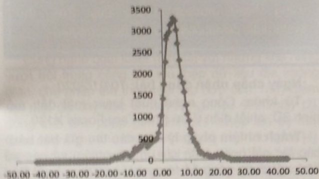
H.4. Biểu đồ tần suất xuất hiện của độ lệch giữa DTU15GRAV so với số liệu đo trực tiếp bằng tàu
