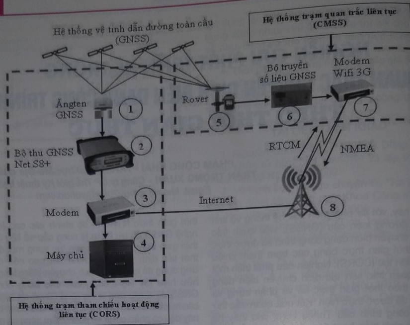
H.1. Sơ đồ hệ thống trạm quan trắc liên tục dịch chuyển biến dạng công trình
