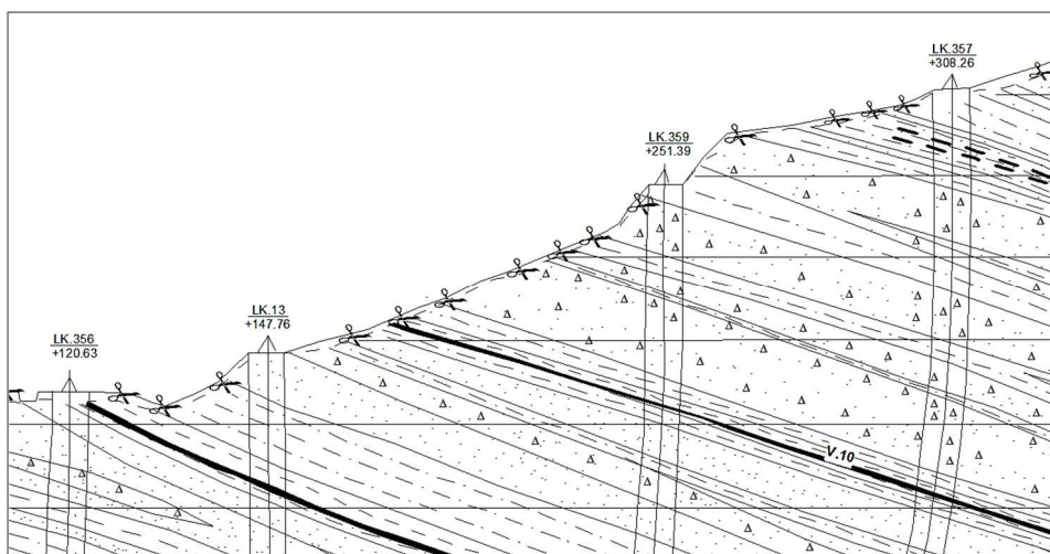
Hình 2. Mặt cắt địa chất tuyến IV.
