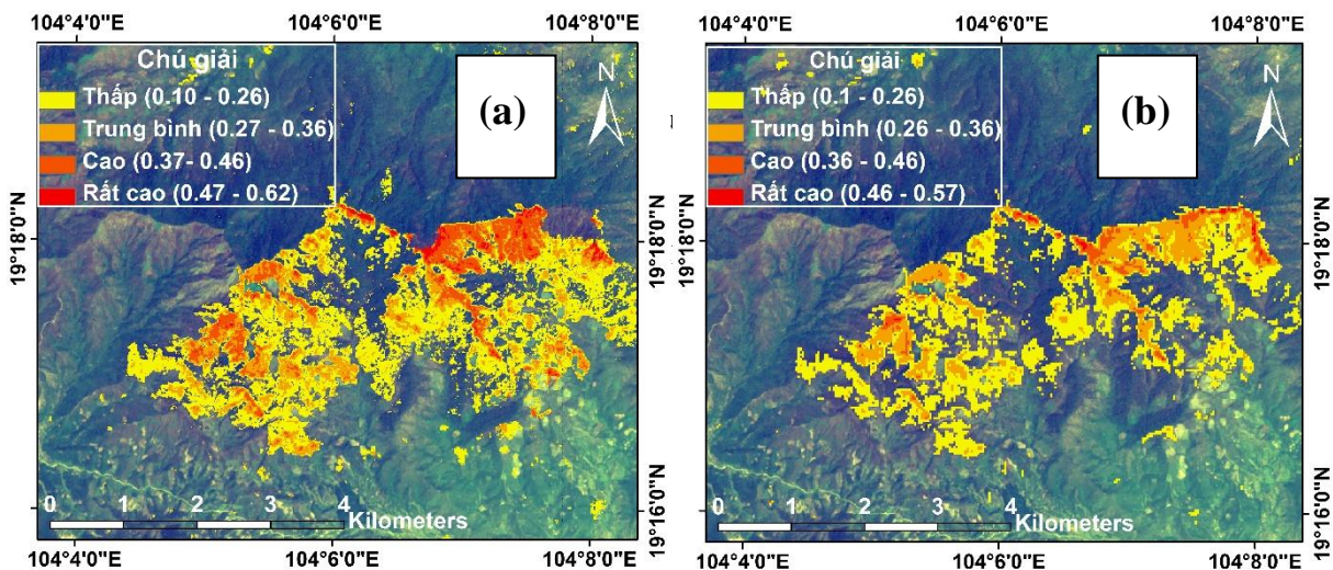
Hình 4. Bản đồ mức độ cháy rừng: (a) thành lập từ ảnh Sentinel-2, (b) thành lập từ ảnh Landsat-8
