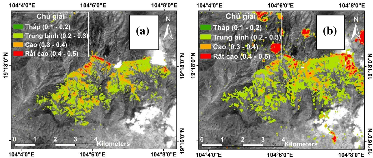
Hình 5. Bản đồ mức độ thay đổi NDVI trước và sau cháy: (a) từ ảnh Sentinel-2, (b) từ ảnh Landsat-8
