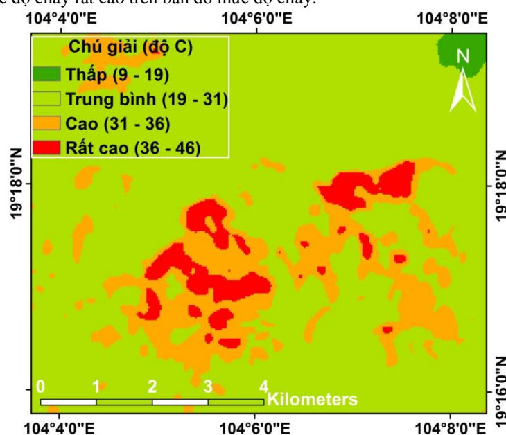
Hình 6. Nhiệt độ bề mặt đất thời điểm xảy ra cháy ngày 20-3-2016 tính từ kênh 10 của ảnh Landsat-8
