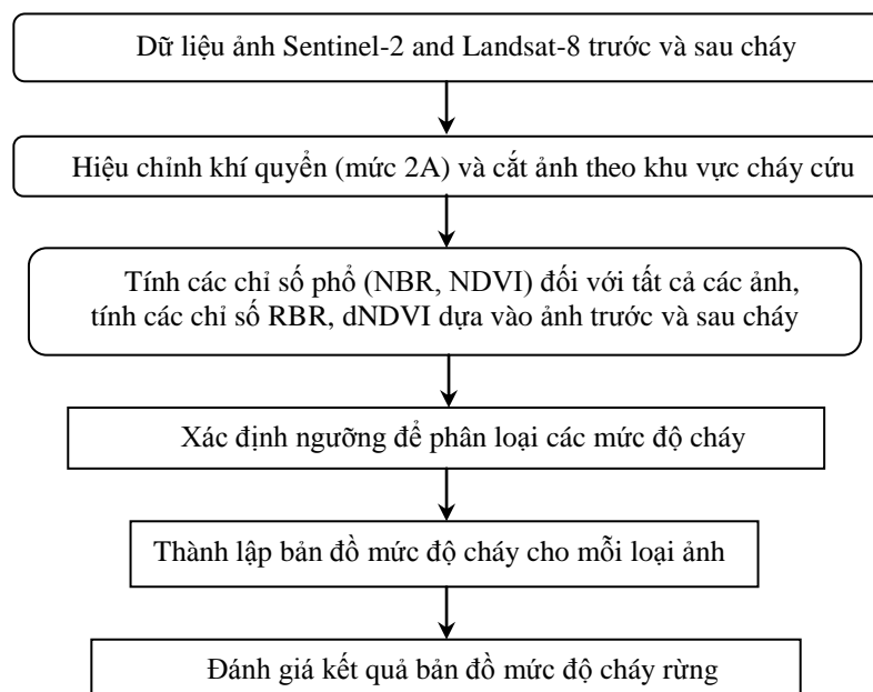
Hình 3. Sơ đồ quy trình thực nghiệm thành lập bản đồ mức độ cháy rừng
