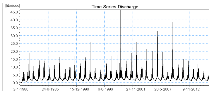
Hình 9. Minh họa diễn biến lưu lượng của 6 mạch lộ được mô phỏng bằng mô hình toán thuộc tỉnh Đắk Nông từ năm 1980 -2016.
