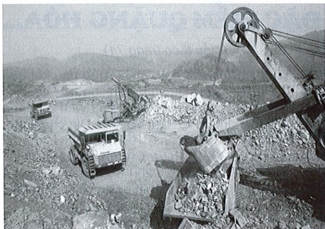
Ảnh 3. Máy khoan TAMROCK và máy xúc điện gầu ngược [7]
