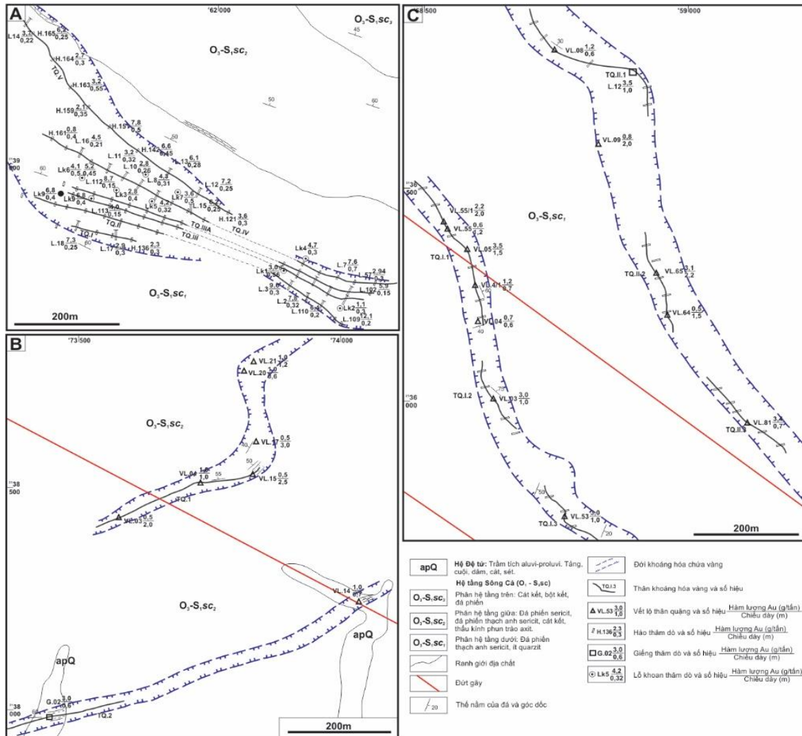
Hình 2. Sơ đồ địa chất và phân bố khoáng hóa vàng khu vực Yên Na - Yên Tĩnh (A) (Trần Văn Thụ và nnk, 2010); Na Khố (B) và Bản Bón (C) (Lê Như Lợi và nnk, 2010).
