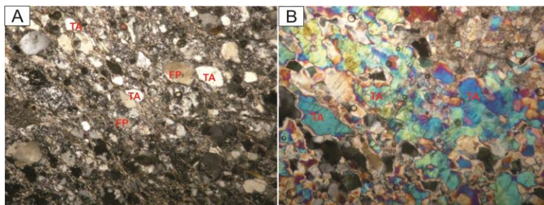
Hình 6. A - đá biến chất động lực điển hình có kiến trúc cà nát (kataclisit), đôi chỗ đến trình độ milonit; B - đới mạch thạch anh nhiệt dịch bị cà nát dập vỡ mạnh (phân tích tại Phòng thí nghiệm Bộ môn Tìm kiếm - Thăm dò, 2017).
