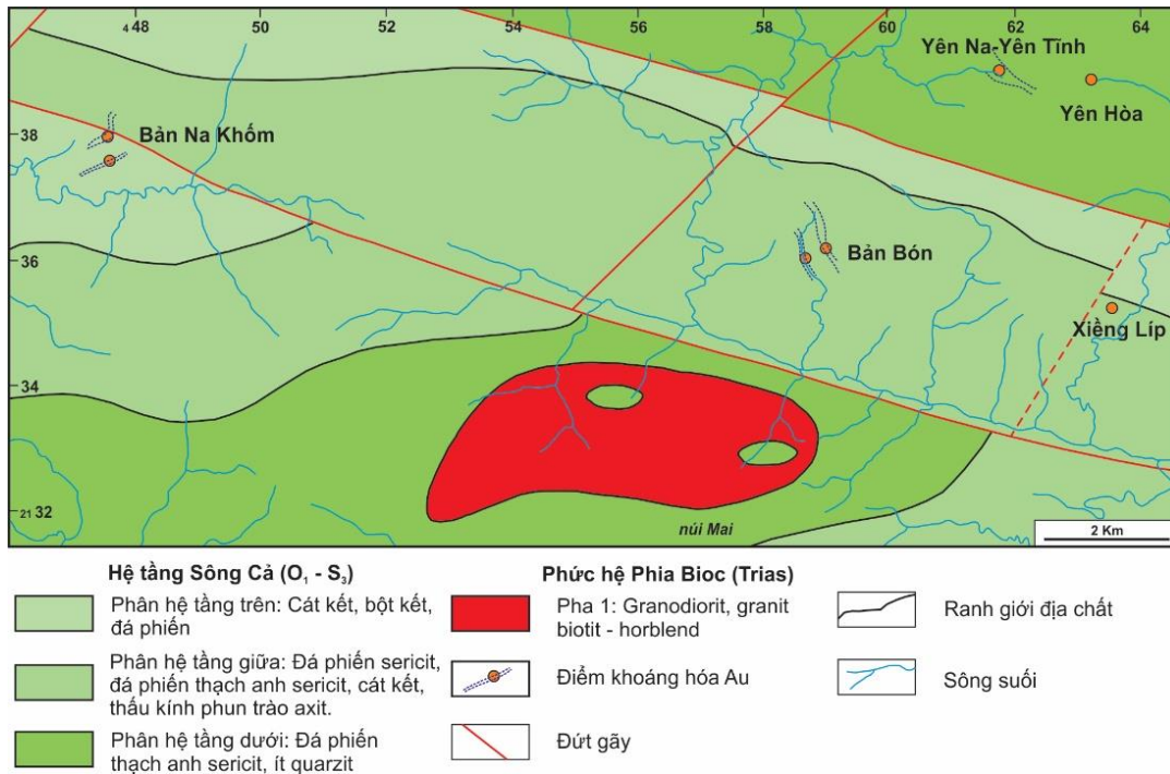
Hình 1. Sơ đồ địa chất khu vực Tương Dương, Nghệ An và vị trí các điểm khoáng hóa vàng (Nguyễn Văn Hoành và nnk., 1994; Trần Toàn và nnk., 1998)
