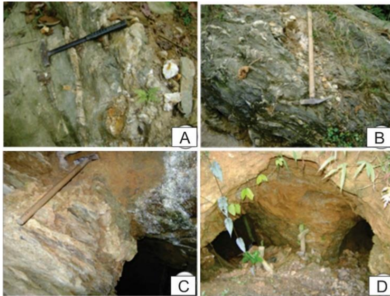
Hình 3. Vết lộ quặng vàng ở khu vực Bản Bón; A, B - thân quặng TQ.I.1, TQ.I.2 được phân bố trong đới mạch thạch anh sulphur chứa Au, màu trắng xám, nâu vàng loang lổ; C, D - thân quặng TQ.II.1, TQ.II.2 trong đới mạch thạch anh chứa vàng màu trắng đục, ám khói có nhiều hang hốc (ảnh Nguyễn Văn Quang trong Lê Như Lợi và nnk., 2010).
