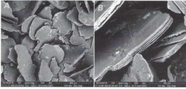
H.2. Hình thái tinh thể graphit vảy tại mỏ Yên Thái huyện Văn Yên tỉnh Yên Bái theo kết quả phân tích điện tử quét (SEM)
